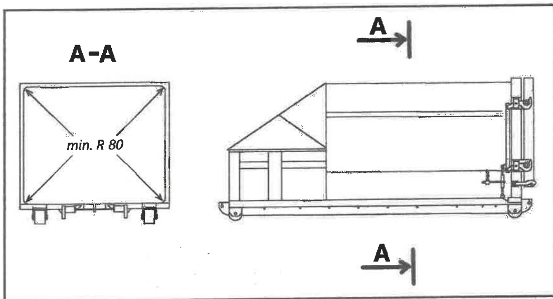
A tömörítőtartályt határoló hosszanti felületeinek belső kapcsolódásánál elvárt min. 80 mm-es rádiusz helyzetét bemutató sematikus rajz.
