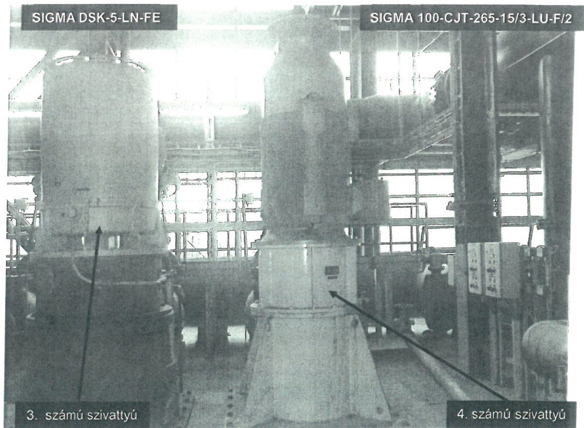
9. számú kép: 3. és 4. számú hűtővíz szivattyúk
