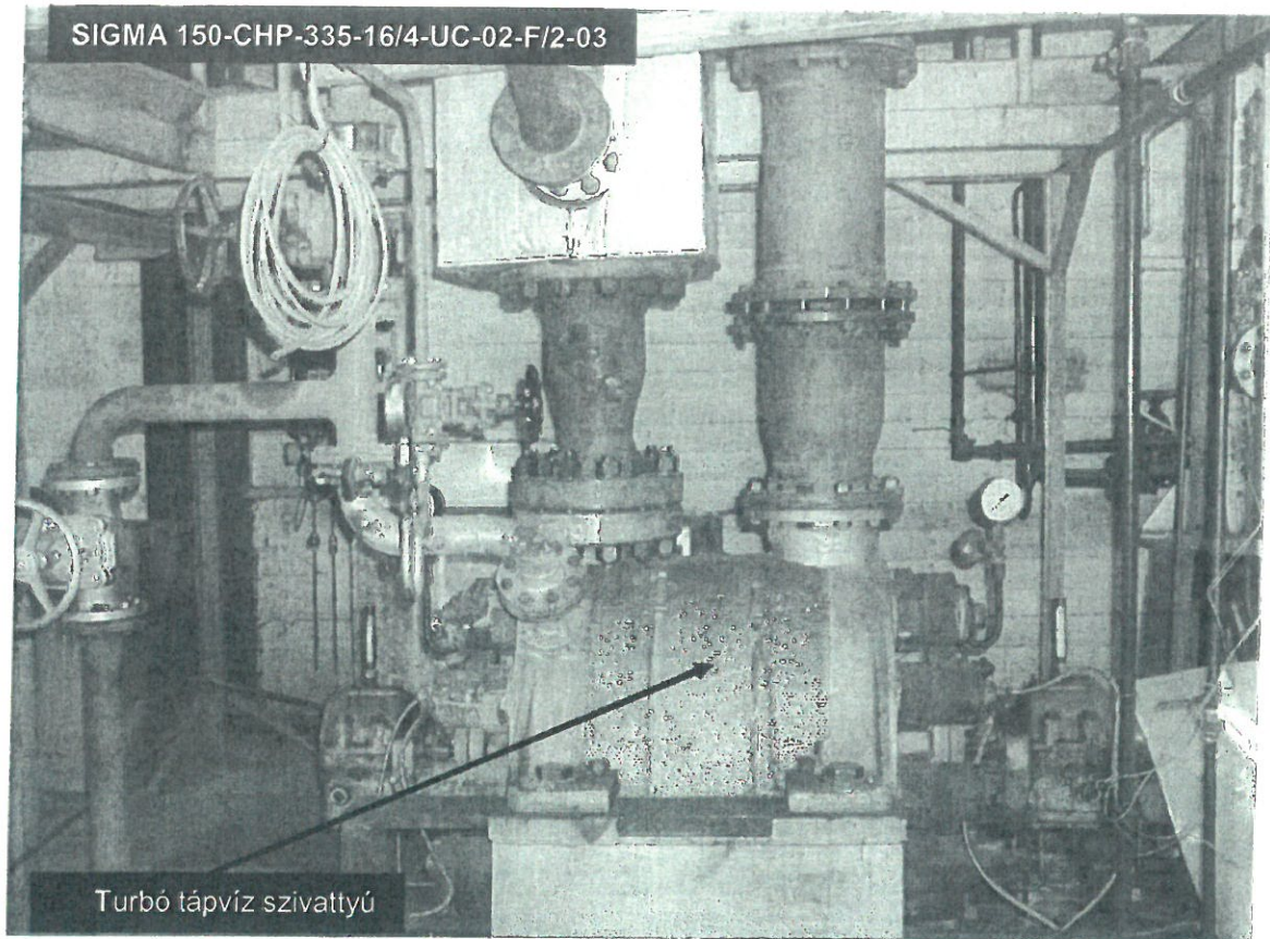
4. számú kép: Turbó tápszivattyú
