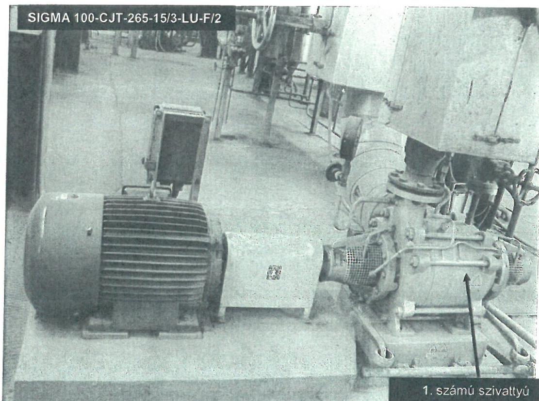
5. számú kép: Szükségkondenzátor 1. számú kondenzátum szivattyú
