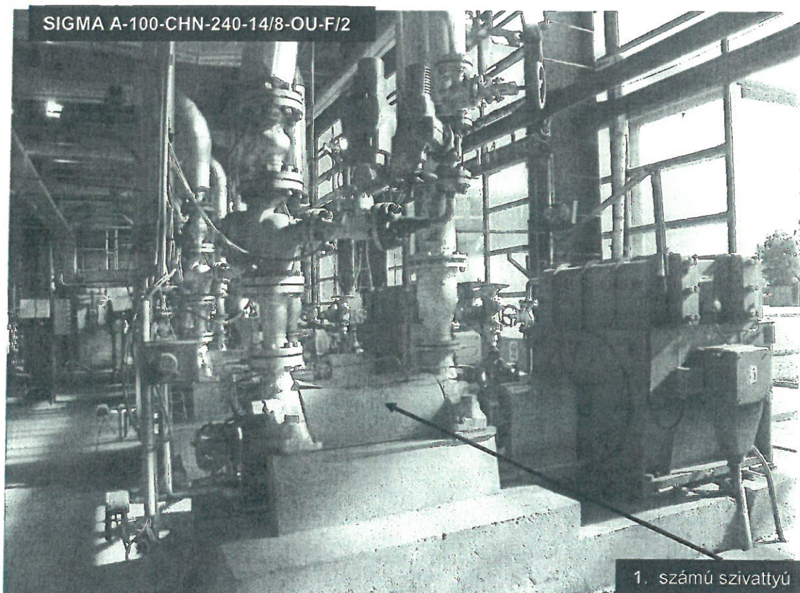
1. számú kép: 1. számú tápszivattyú
