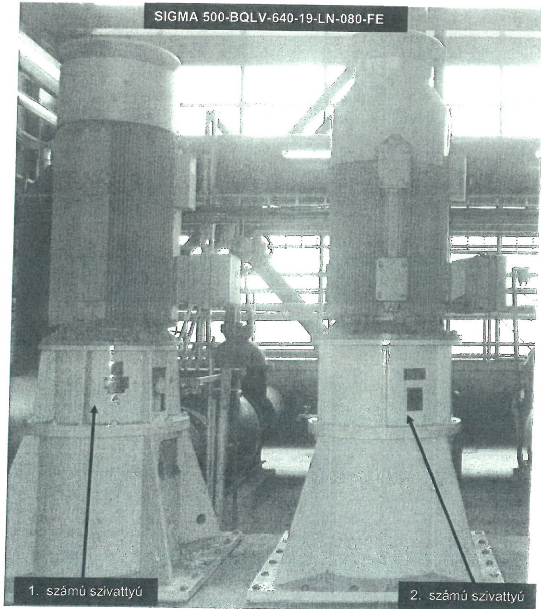
8. számú kép: 1. és 2. számú hűtővíz szivattyúk
