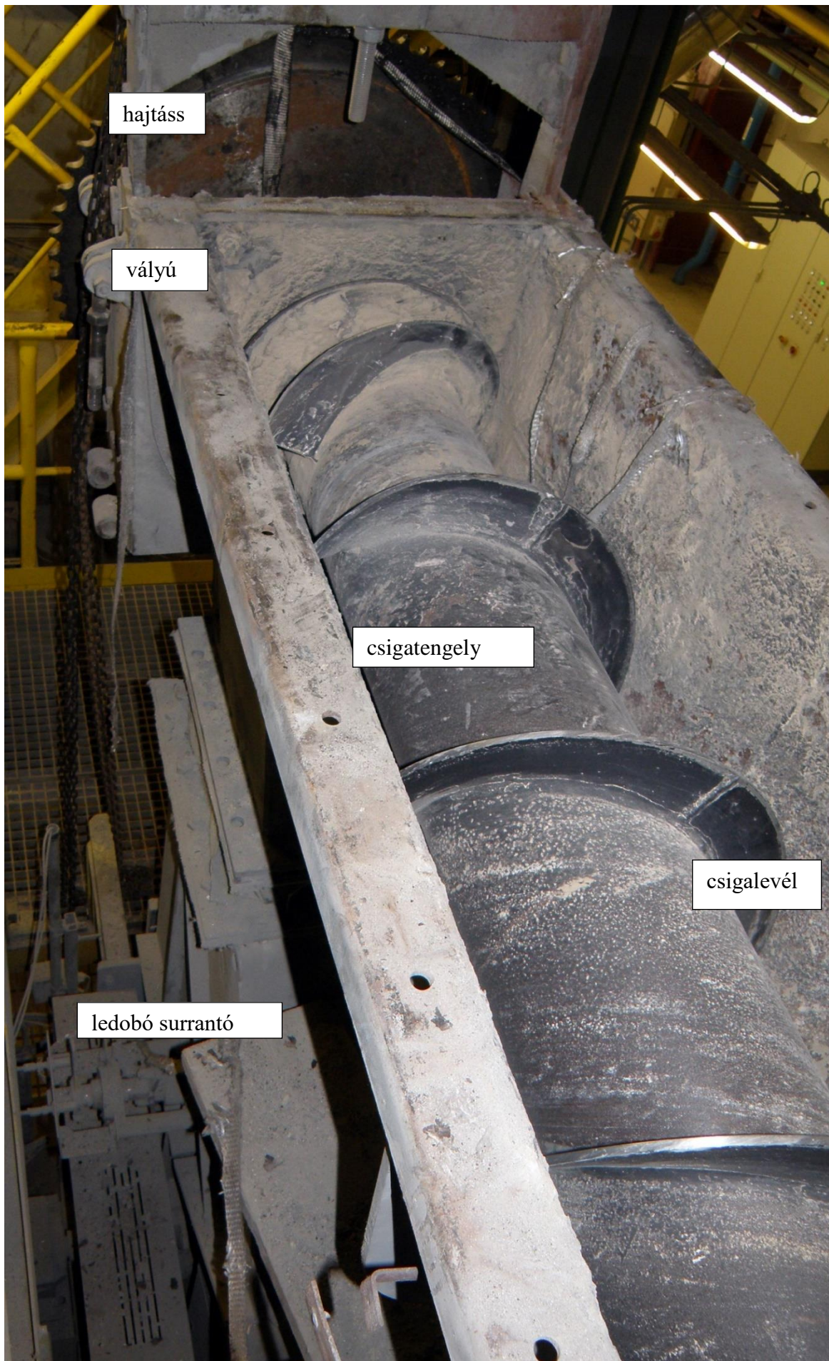
3. kép: a megbontott berendezés hajtás felőli vége, vályú és csiga
